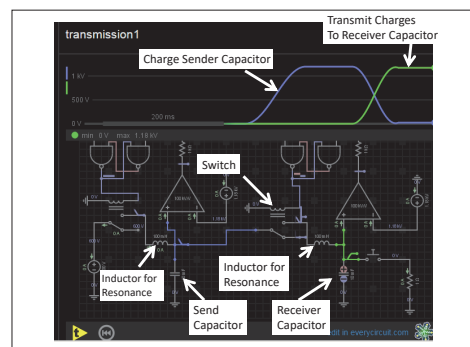
電力パケットネットワークのシミュレーション Simulation of electric power packet networking
