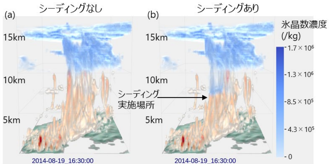
図 3. シーディングによる線状降水帯の 3 次元構造の変化。
