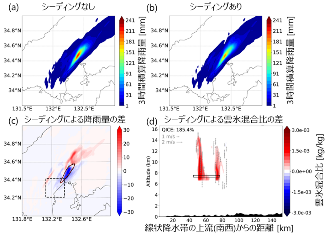
図 2. シーディングによる線状降水帯の降雨量の変化。
