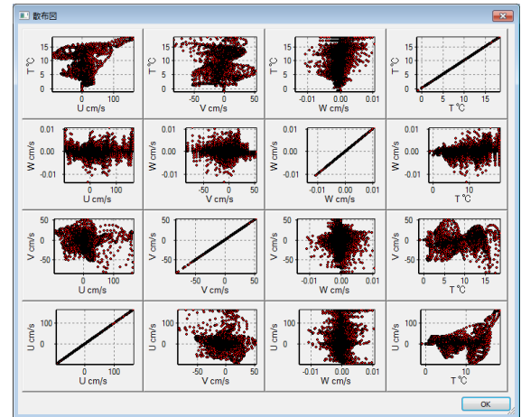
変数空間
