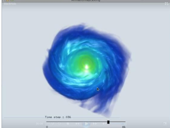
ブラックホールシミュレーション (木内先生@京都大学)
