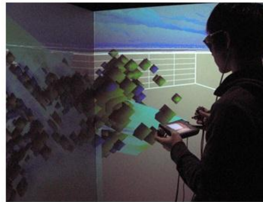
新潟中越地震の震源分布(断層面の推定)
