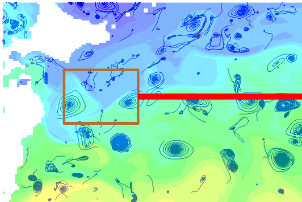
座標空間
