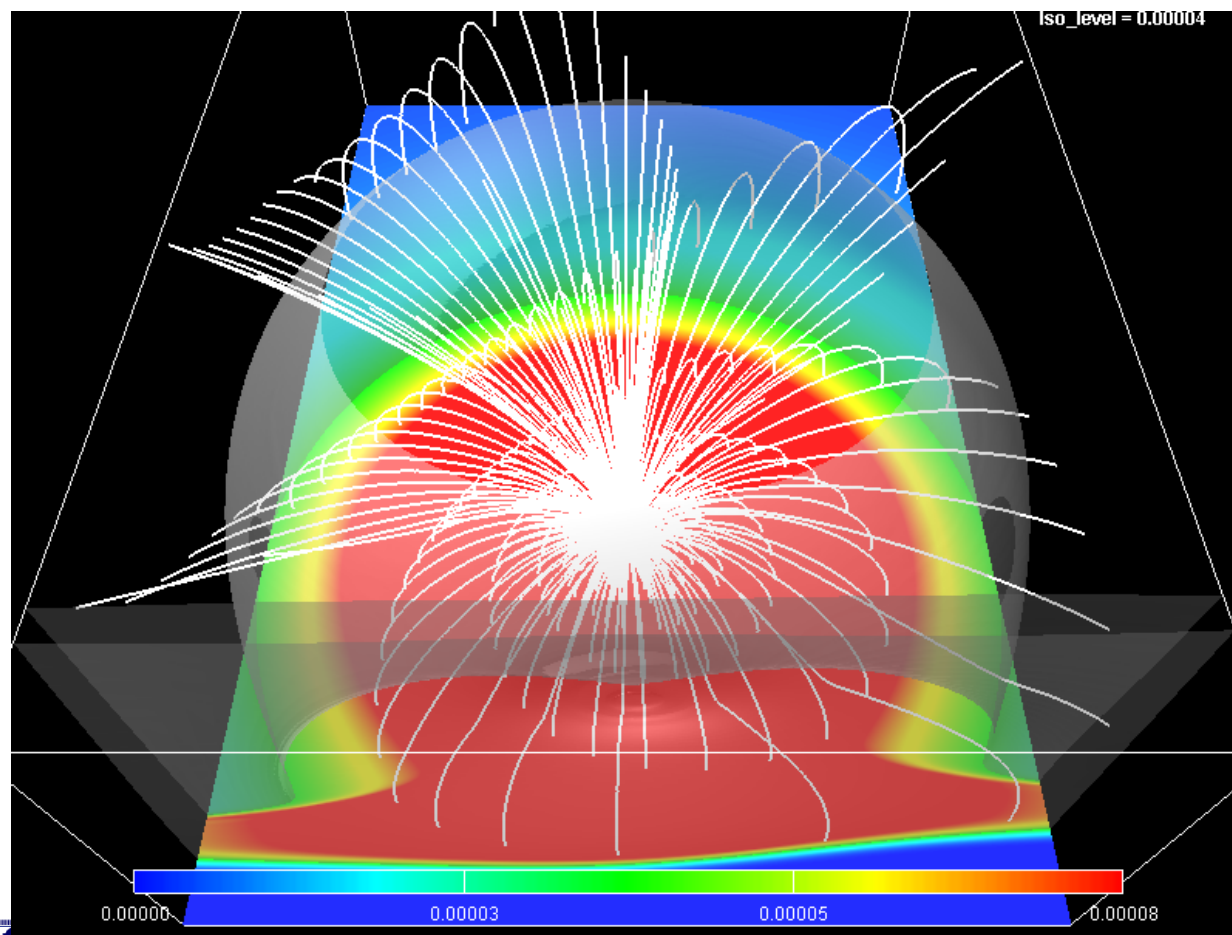
Fig. 土星磁気圏赤道面における磁場強度[Fukazawa et al., JGR, 2012]
